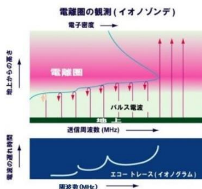
図2 イオノグラムの原理
